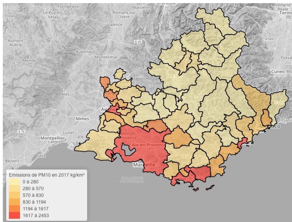
Figura 24 - Inventario delle emissioni della Regione Provence-Alpes-Côte d'Azur 2017: distribuzione spaziale delle emissioni totali di PM 10
