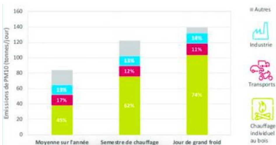
Figura 21 - Inventario delle emissioni della Regione Auvergne-Rhône-Alpes 2015: contributo dei settori alle emissioni di PM 10 in differenti periodi dell'anno
