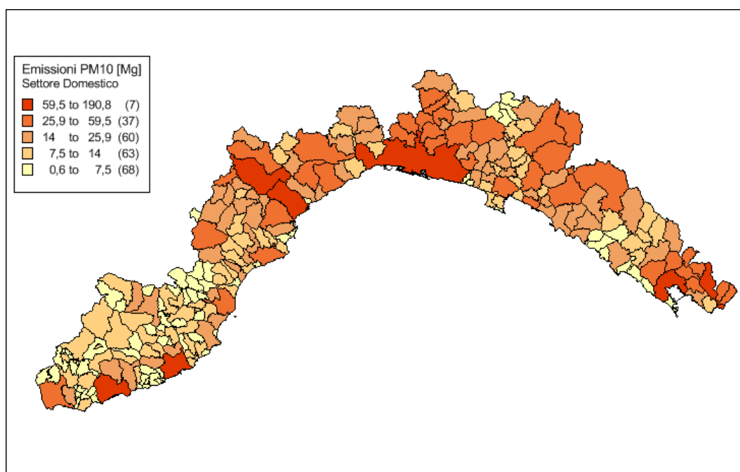
Figura 15 – Regione Liguria - Emissioni totali di PM 10 (Mg) nel settore residenziale – Anno 2016
